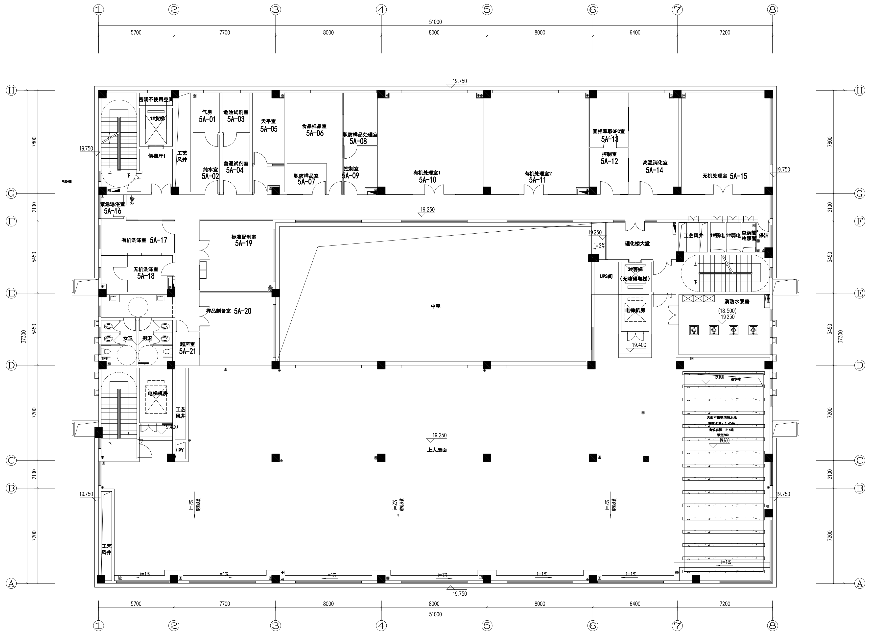
五层平面布置图 1:100
